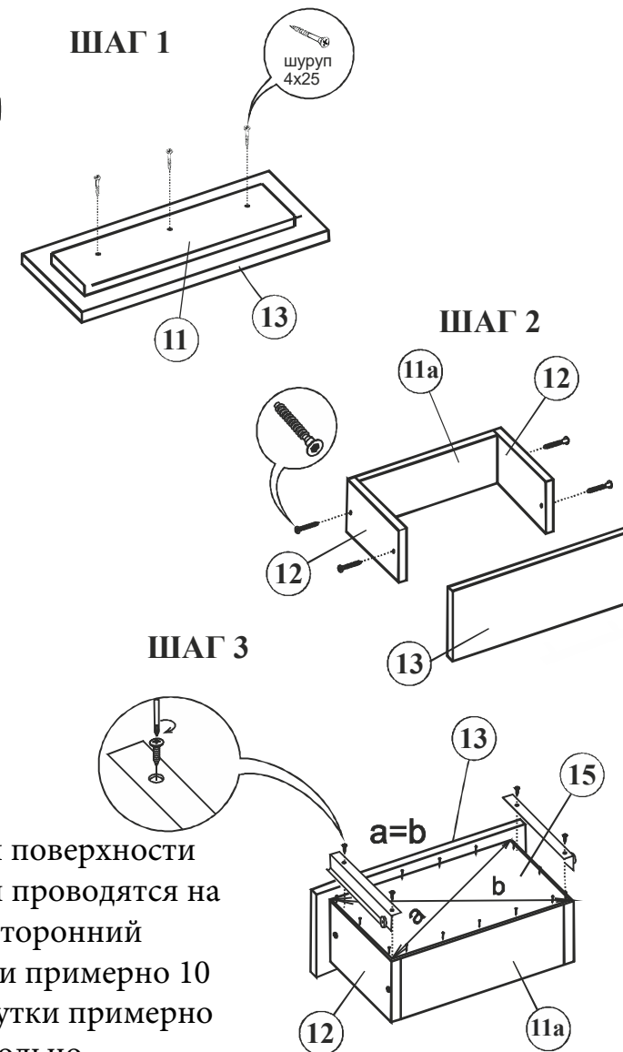
Рис.3 Порядок сборки выдвижного ящика
