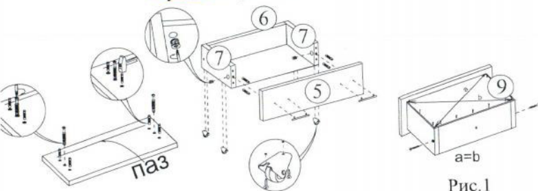
Порядок сборки выдвижного ящика
