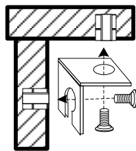
Схема установки стяжки угловой
