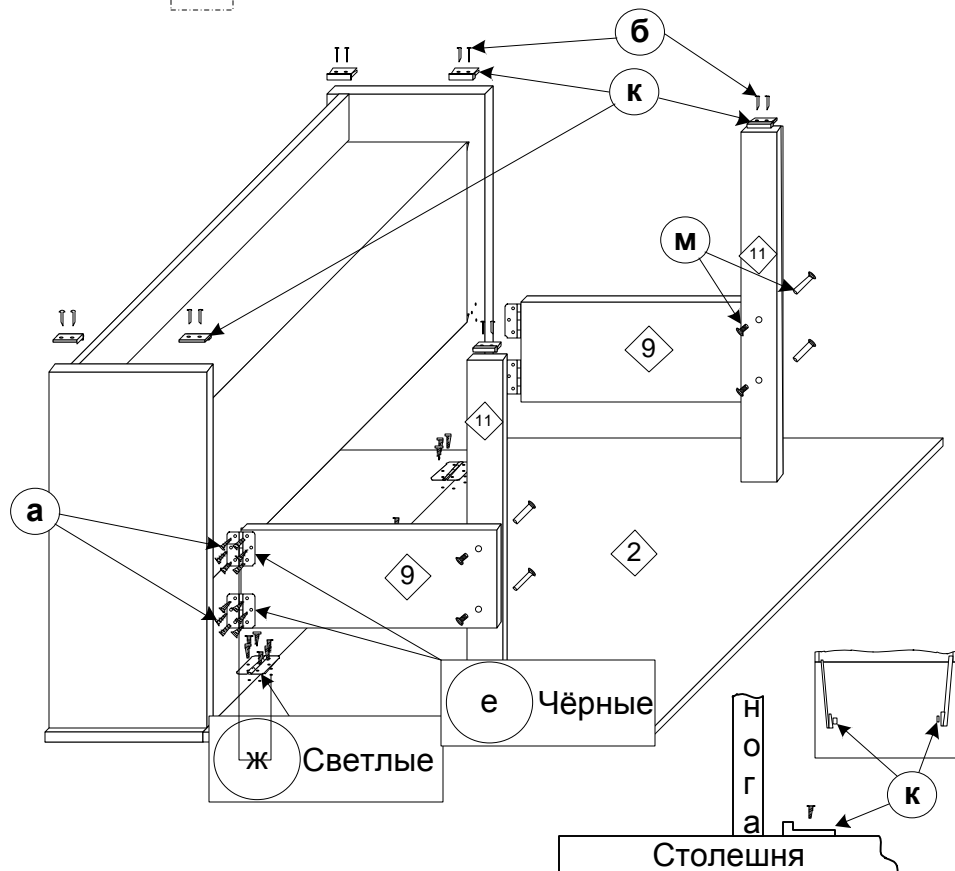
2 Схема установки опор и столешни
